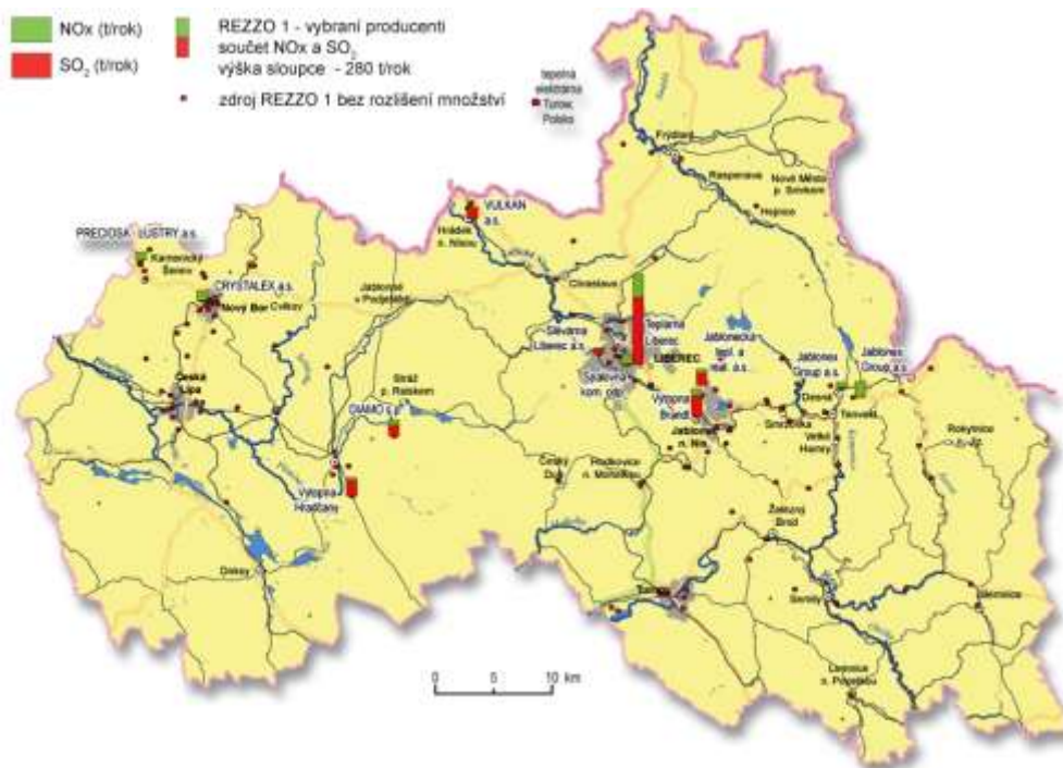
Obrázek 16: Bodové zdroje na území Libereckého kraje dle REZZO
