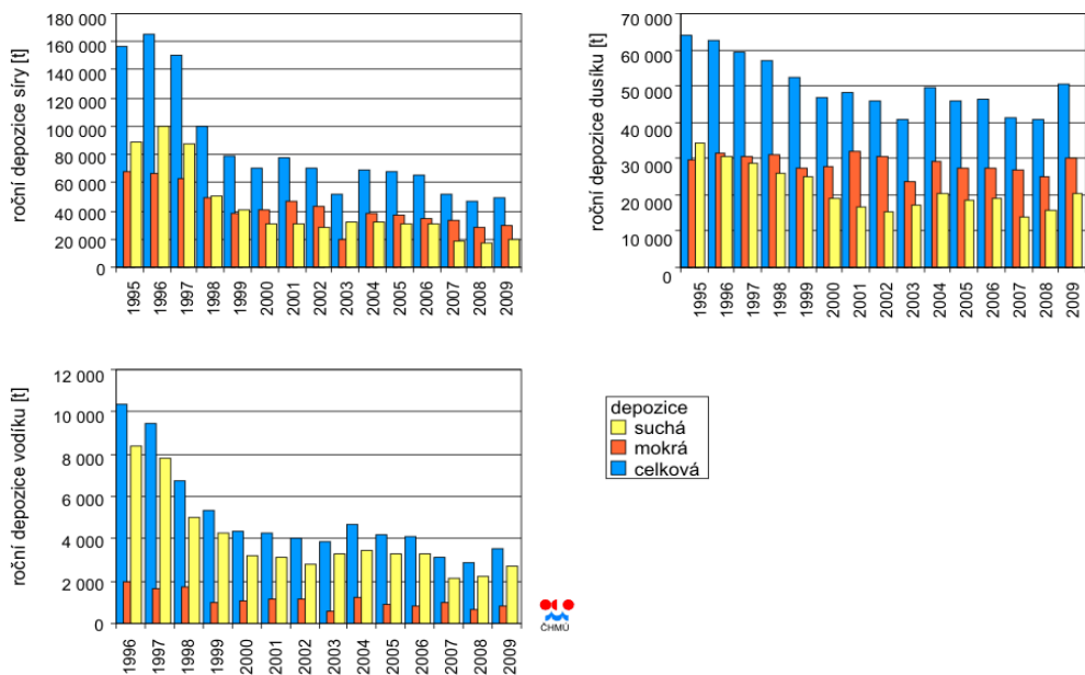
Obrázek 17: Dlouhodobý vývoj depozic imisí na území ČR
